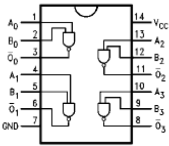
74AC00
