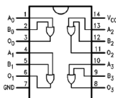
74AC32
