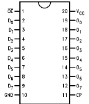
74AC574
