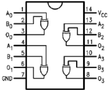
74AC86
