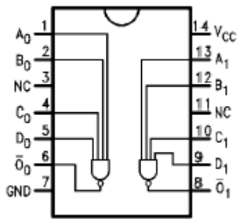
74AC20
