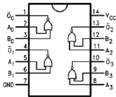
74AC02
