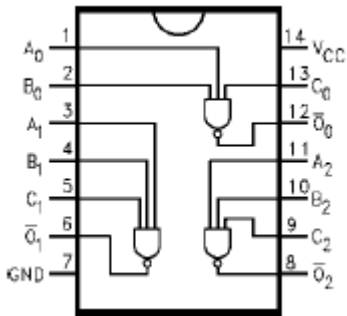
74AC10
